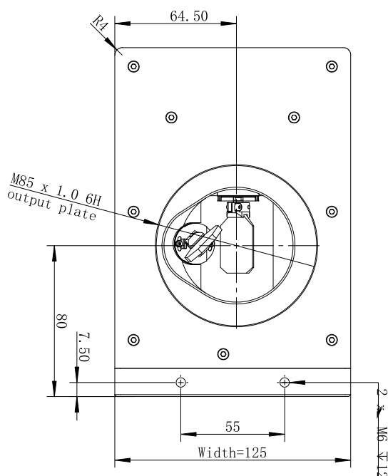
外形尺寸图
